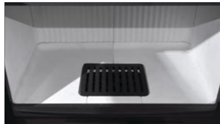
BELLANO, chambre de combustion doublée en thermo-béton blanc.
